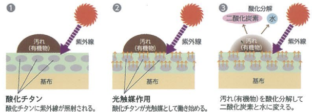
光触媒防汚メカニズム
